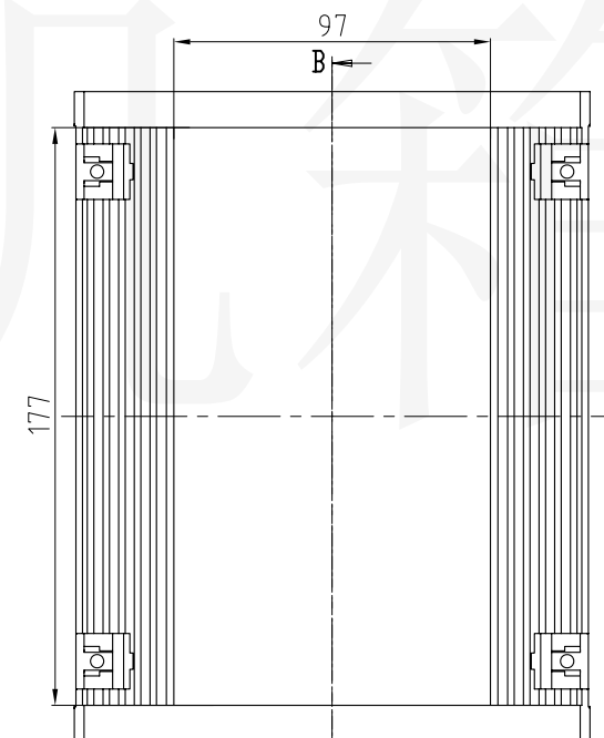
B 装配体
